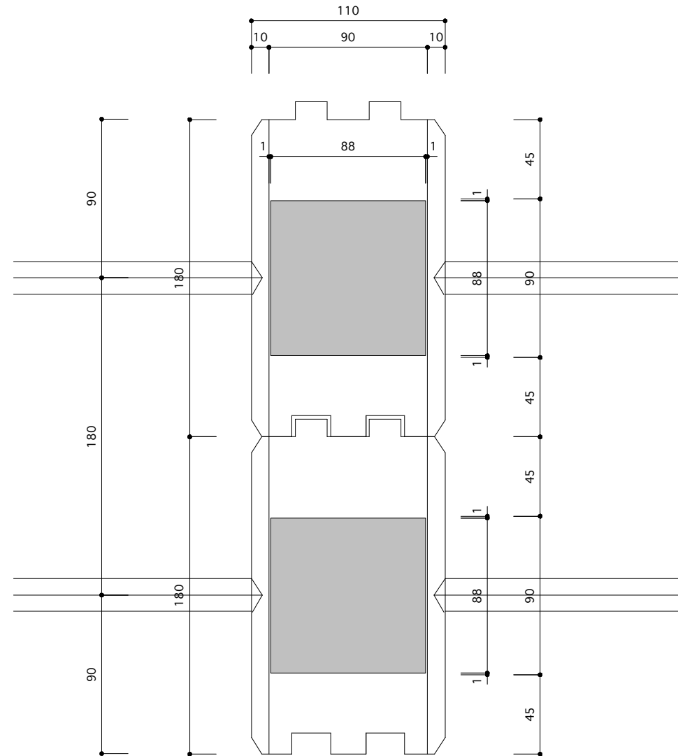
ログ断面詳細 S=1/3
