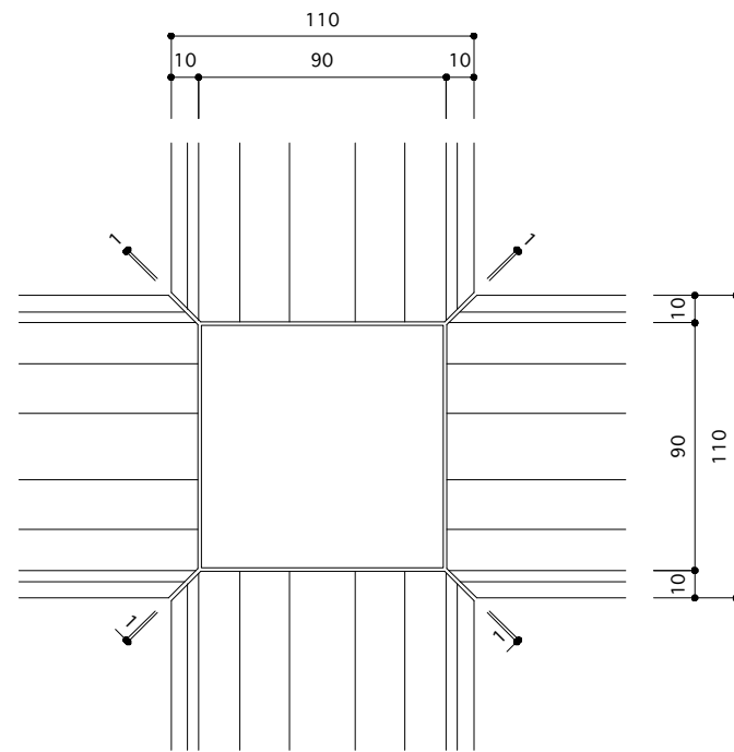
ログ断面詳細 S=1/3
