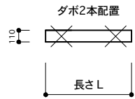
L=810 / 土台
