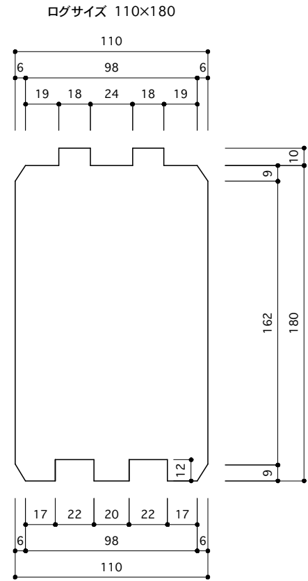
ログ断面詳細 S=1/3
