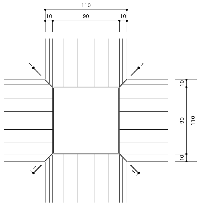
ノッチ平面詳細 S=1/3
