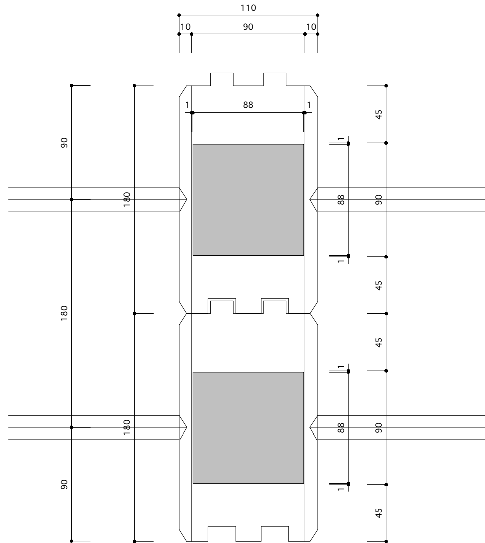
ノッチ断面詳細 S=1/3
