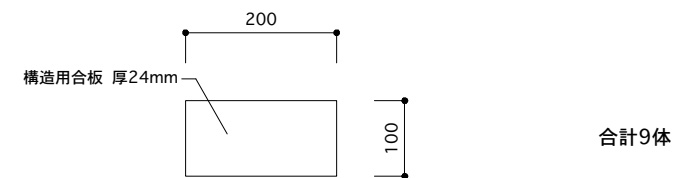
層間変位測定用 木製架台パーツ3 S=1:10
