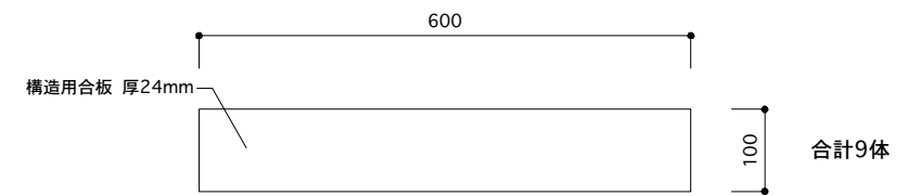
層間変位測定用 木製架台パーツ2 S=1:10
