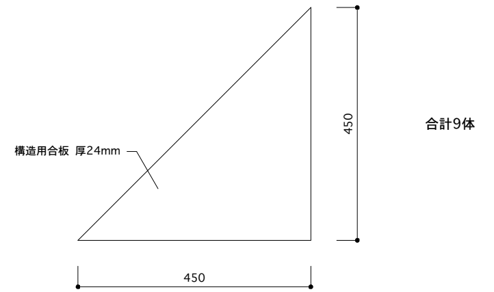
層間変位測定用 木製架台パーツ1 S=1:10
