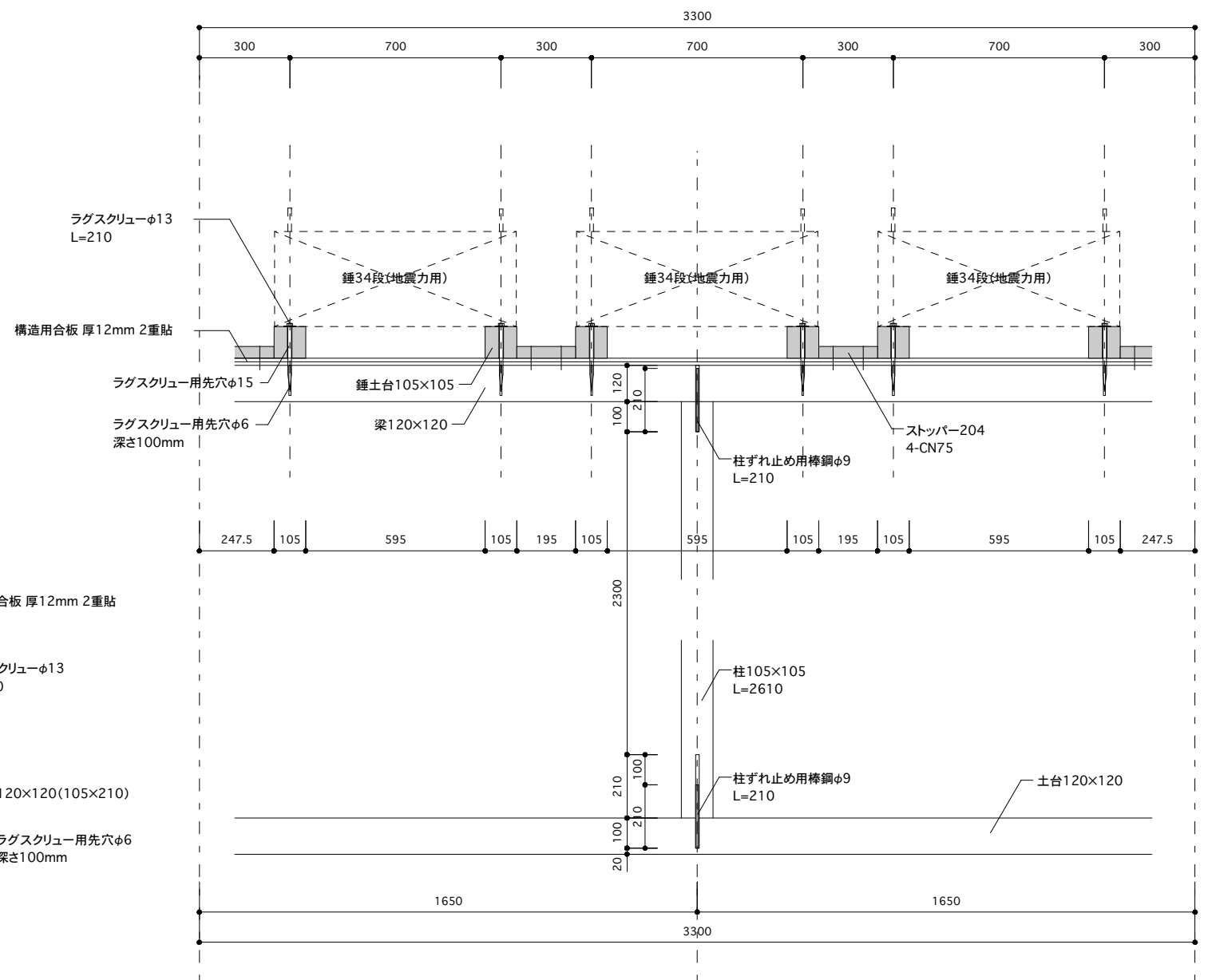
錘土台詳細図(地震力用錘) S=1:20
