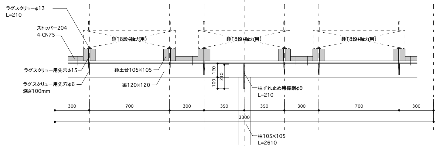
錘土台詳細図(軸力用錘) S=1:20
