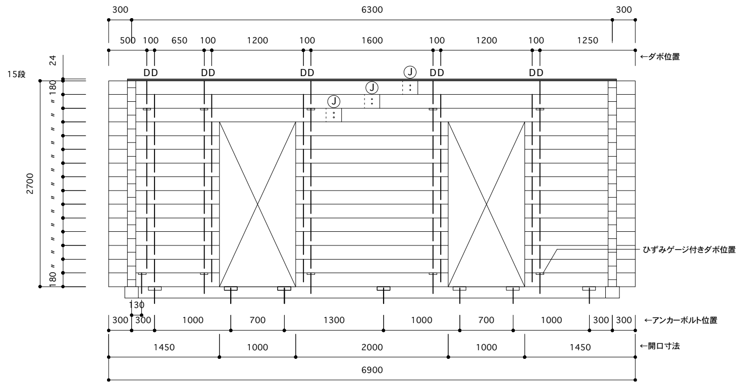
すだれ壁試験体(L=2000)・壁見附図
