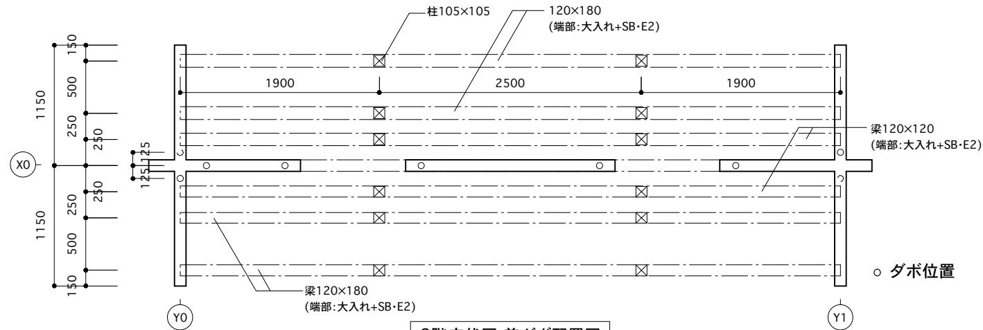
2階床伏図 兼ダボ配置図
