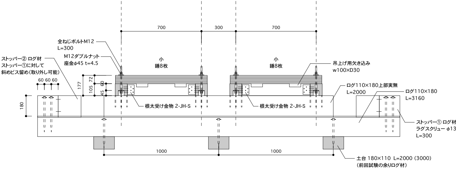
L=2000試験体 S=1:20
