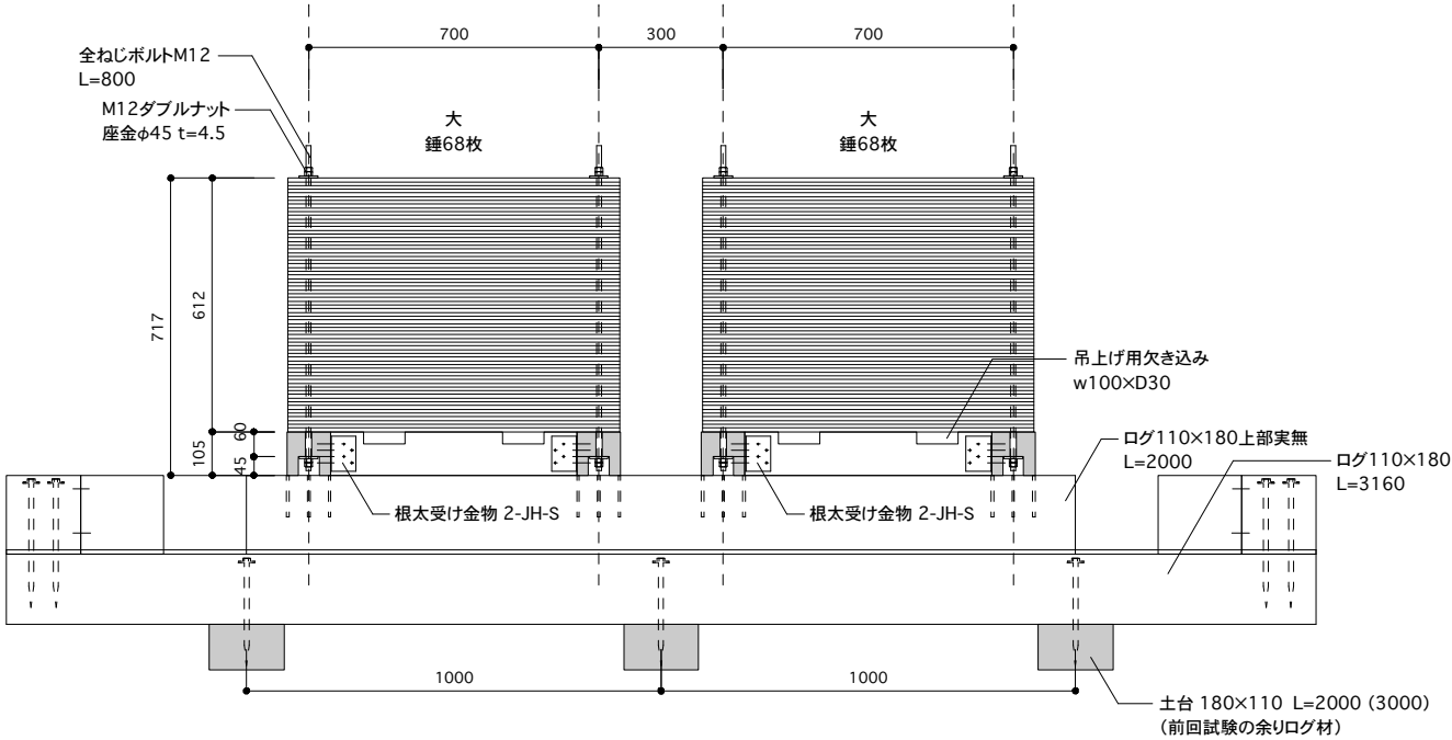
L=2000試験体 S=1:20
