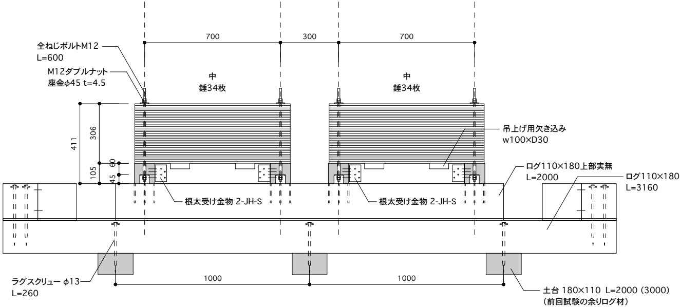
L=2000試験体 S=1:20
