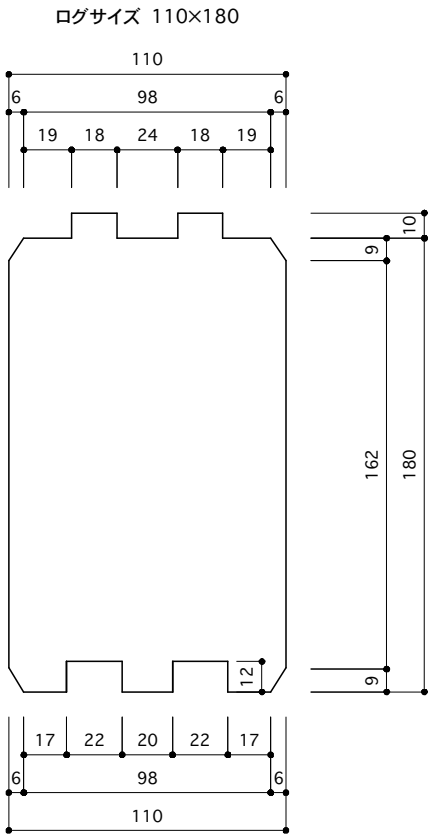
ログ断面詳細 S=1/3
