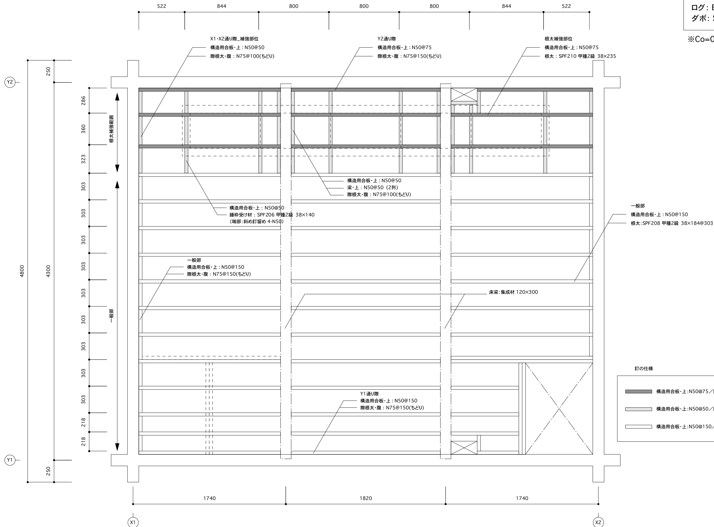
釘仕様詳細図 S=1/50
